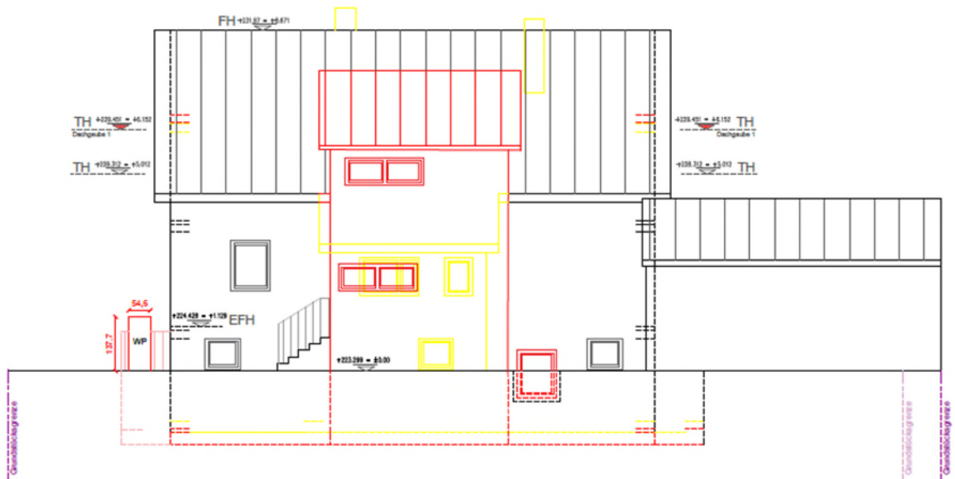
Ansicht Ost
