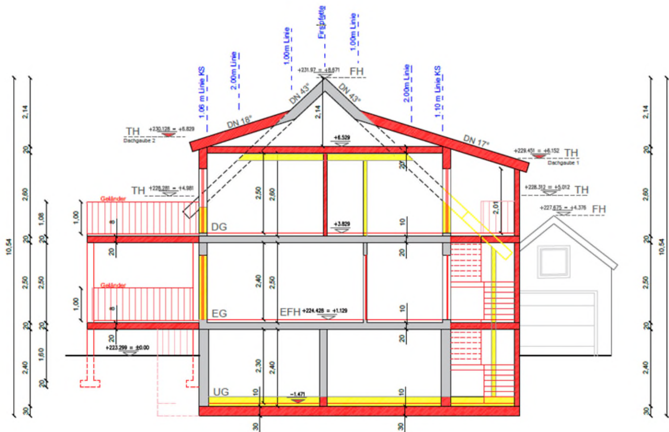
Schnitt A-A
