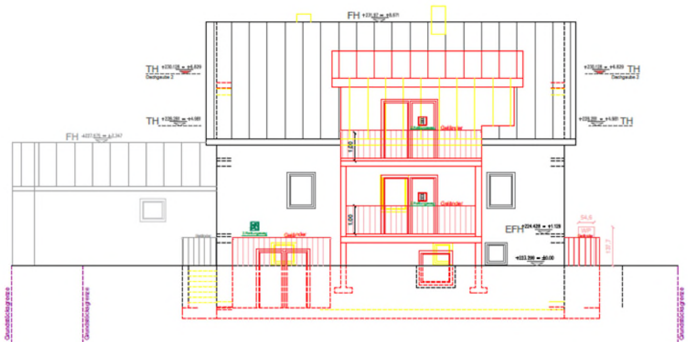
Ansicht West
